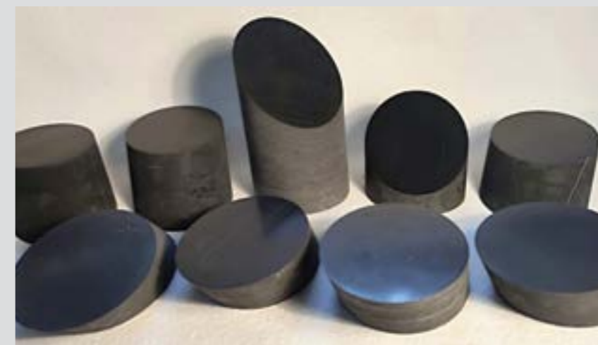
Vzorky vrtných jadier priemeru 60 mm z hĺbky cca 40 (!) metrov z realizovaného vrtu v rámci inžinierskogeologického a hydrogeologického prieskumu pre stavbu diaľnice D4 Bratislava-Záhorská Bystrica.
